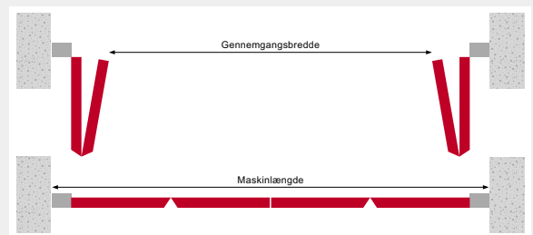
Plan snit (montering mellem vægge)
