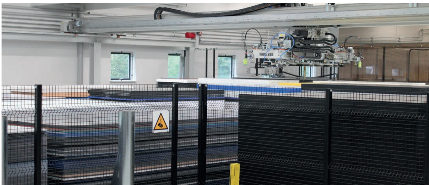
Hurtig klargøring af materialer: Vores fuldautomatiske pladelager er direkte forbundet til en 5-akset fræser.
