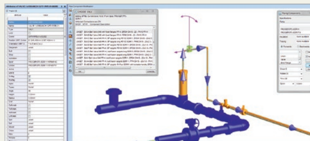
AVEVA PLANT PDMS 3D piping using PROGEF catalog data
