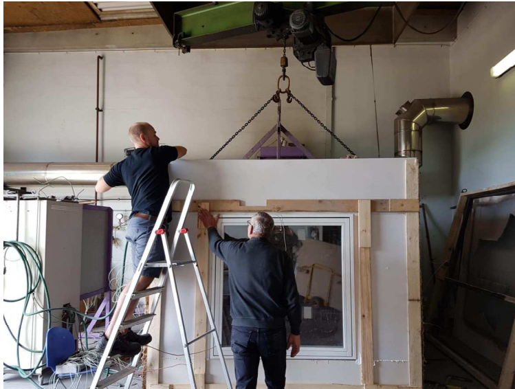
Beklædning foran isolering på test element ( for at holde på varmen )
