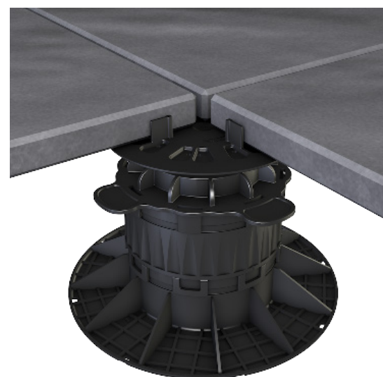
SemiFix PRO justerbar flisefod
