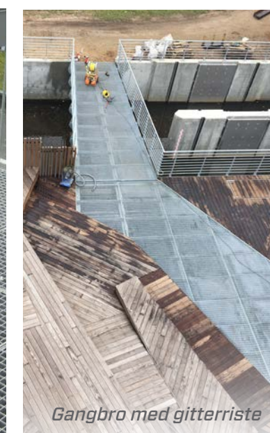
Gitterriste som platform
