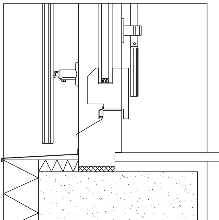
Snittegning med drejestangsbetjening
