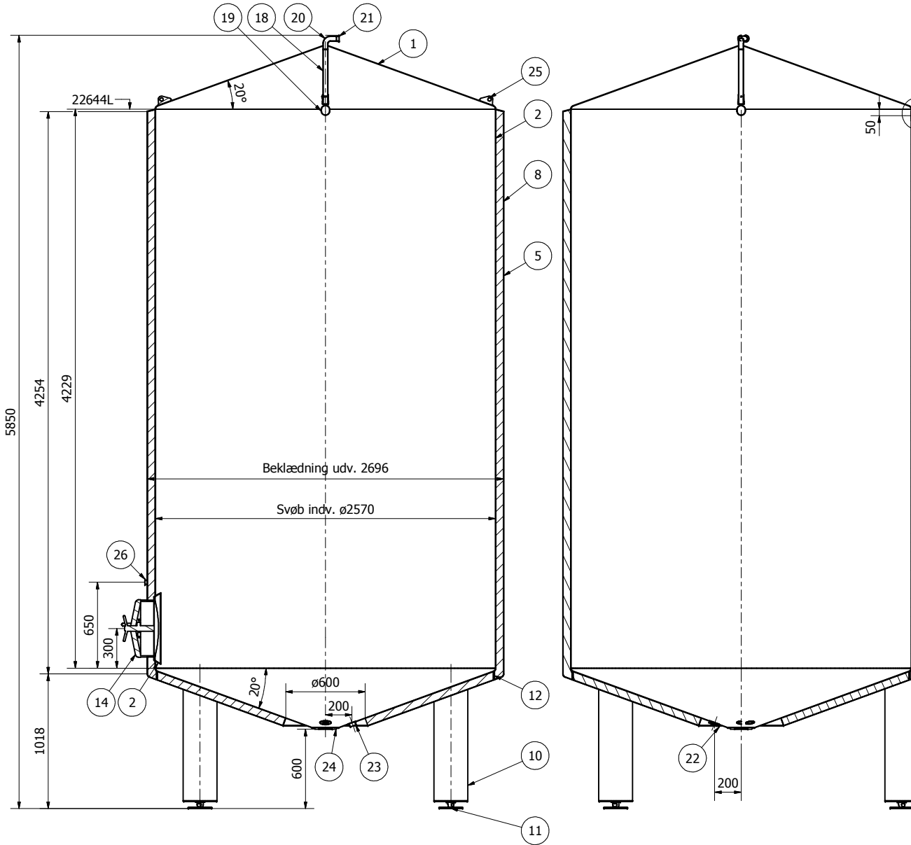
B-B ( 1 : 20 )
