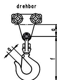
Med svirvel- lastkrog
