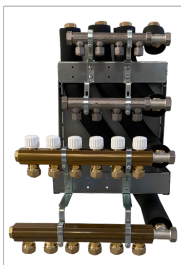
BUNDMODUL med 6 gulvvarme-, 4 koldtvands- og 4 varmtvandskredse.
