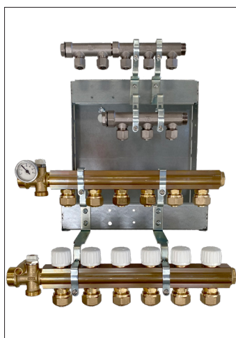
Standard skaktløsning med 5 eller 6 gulvvarme-, 5 koldtands- og 3 varmtandskredse.
