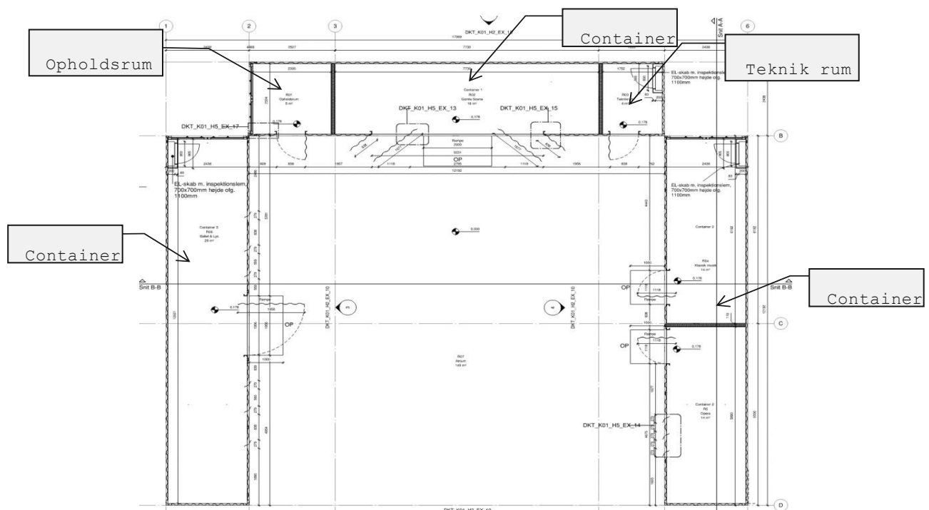
Figur 1: Planopstilling med tre containere, som danner en udendørs atriumgård
