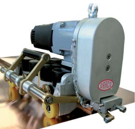
Elektrisk falsemaskine K9-1, - den rette falsemaskine til stående enkelt- eller dobbeltfals.
