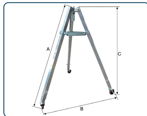
Måttskiss WIMAG trebock. Bilden visar D-250 mobil
