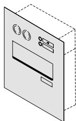
Frontplade 2 mm Galfan-stål eller rustfrit stål V4A
