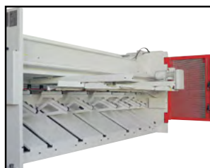
Pneumatisk pladefang type A
