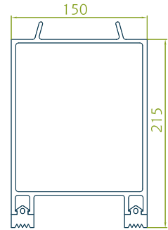
PROFIL 150/215 váha 10,30 kg/m
