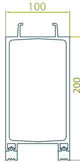
PROFIL 100/200 váha 8,70 kg/m
