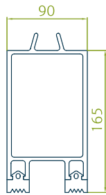
PROFIL 90/165 váha 6,70 kg/m
