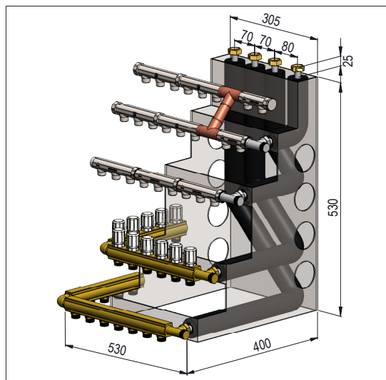
Max. bestykning af et BUNDMODUL for at det kan være i et 60 cm skab. 12 gulvvarme-, 16 koldtands- og 9 varmtvandskredse.
