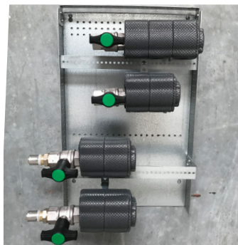
Max. bestykning af et BUNDMODUL for at det kan være i et 60 cm skab. 12 gulvvarme-, 16 koldtands- og 9 varmtvandskredse.
