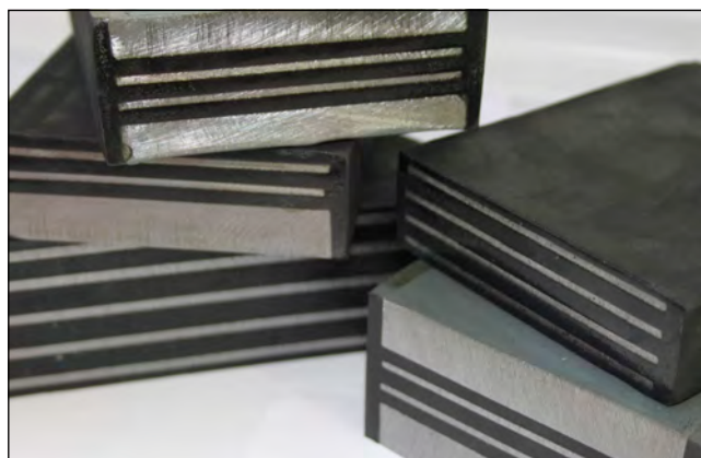
AAG bæreløjer
