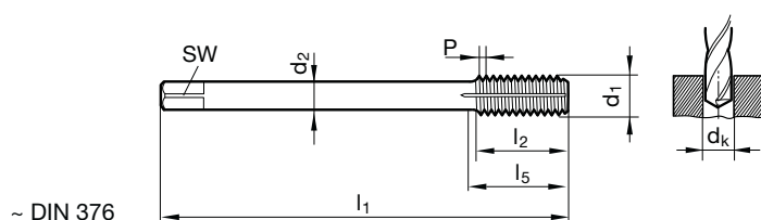
~ DIN 376
