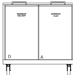
BE-550-3 Miljövägn på hjul. Innehåll 2st lådor. B 820 x H 845 x D 650mm. Lådstorlek D x 2st. B 305 x D 615 x H 600mm. Alternativ lådindelning istället för D. Lådstorlek A x 2st. B 305 x D 325 x H 600mm.
