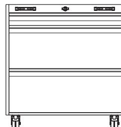
BE-500-Rekond Verktysvägn med 3st lådor. Centrallåsning öppnar en låda i taget. B 820 x H 850 x D 600mm. Lådstorlek x 1 B 755 x H 70 x D 420mm. Lådstorlek x 2 B 755 x H 250 x D 420mm. Modulstorlek B 900 x H 880 x D 660mm.
