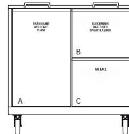
BE-550-7 Miljövägn på hjul. Innehåll 7st lådor. B 820 x H 845 x D 650mm. Lådstorlek A x 2st. B 305 x D 325 x H 600mm. Lådstorlek B x 3st. B 205 x D 325 x H 265mm. Lådstorlek C B 325 x D 545 x H 220mm.
