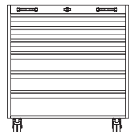
BE-500 Verktysvägn med 6st lådor. Centrallåsning öppnar en låda i taget. B 820 x H 850 x D 600mm. Lådstorlek x 3 B 755 x H 70 x D 420mm. Lådstorlek x 2 B 755 x H 110 x D 420mm. Lådstorlek x 1 B 755 x H 140 x D 420mm. Modulstorlek B 900 x H 880 x D 660mm.
