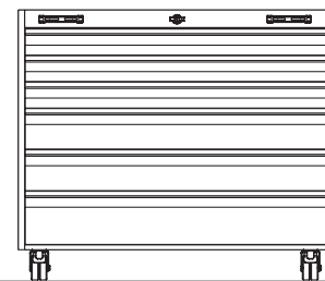
BE-500-XL Verktysvägn med 6st lådor. Centrallåsning för öppning av en låda i taget. B 1010 x H 850 x D 600mm. Lådstorlek x 3 B 970 x H 70 x D 420mm. Lådstorlek x 2 B 970 x H 110 x D 420mm. Lådstorlek x 1 B 970 x H 140 x D 420mm. Modulstorlek B1090 x H 880 x D 660mm.
