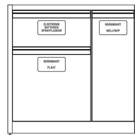
BE-900-3x/MILJÖ Sektion med 2 lådor. Lådstorlek x 1 (3st sorteringskär) B 495 x H 220 x D 600mm. Lådstorlek x 1 (1st sorteringskär) B 495 x H 490 x D 600mm. Modulstorlek B 600 x H 880 x D 660mm.
