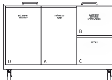
BE-550-XL7 Miljövägn på hjul (bredd: 1275mm). Innehåll 7st lådor. B 1200 x H 845 x D 650mm. Lådstorlek D x 1st. B 305 x D 615 x H 600mm. Lådstorlek A x 2st. B 305 x D 325 x H 600mm. Lådstorlek B x 3st. B 205 x D 325 x H 265mm. Lådstorlek C B 325 x D 545 x H 220mm.
