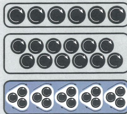
Gruppo spazzole tangenziali / sistema planetario Tangential brushes unit / planetary system Unidad de cepillos tangencial / sistema planetario
