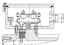
Frame size 132–160
