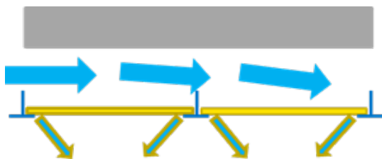
Principperne for diffus ventilation med et nedhængt loft
