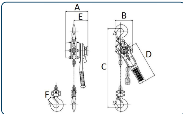
Måttskiss KITO Spaklyftblock LB
