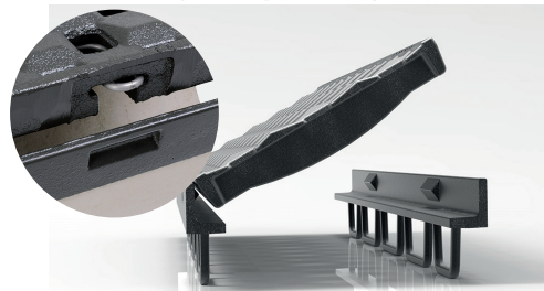
Kliklåsesystem på støbejernsriste
