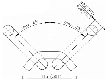
DOUBLE 36 & 50 TON
