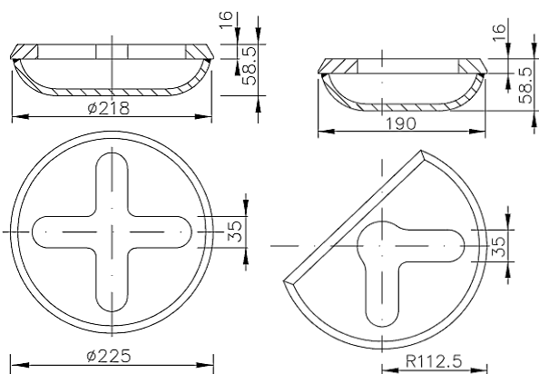
FLUSH
