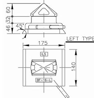
TRANSVERSAL 45°
