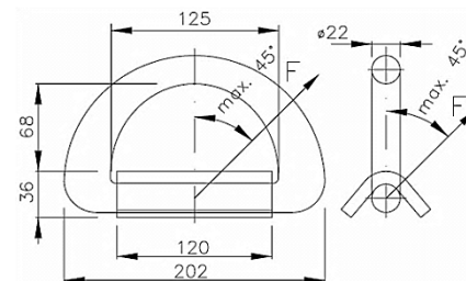
36 TON
