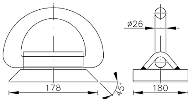
DOVETAIL 45°
