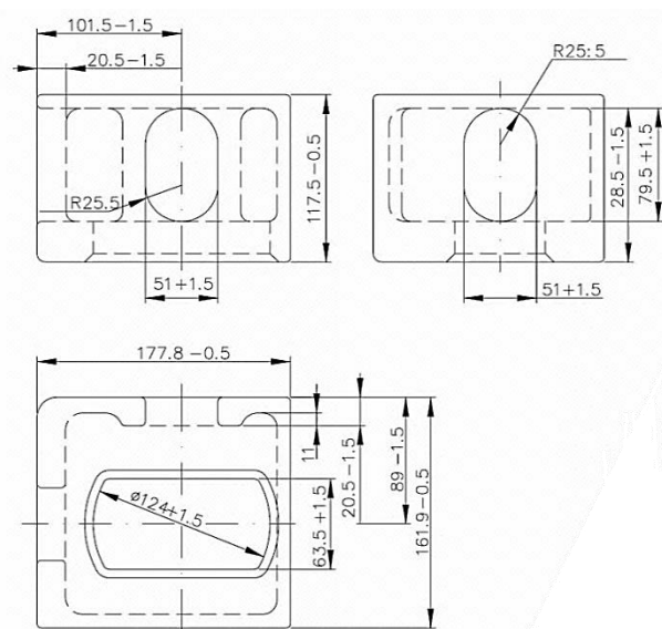
BOTTOM ISO LEFT
