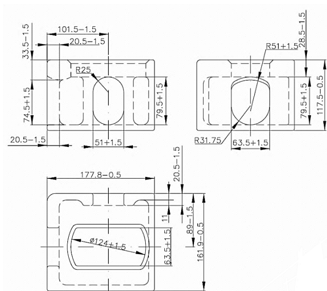
TOP ISO LEFT
