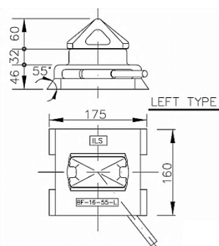
TRANSVERSAL 55°
