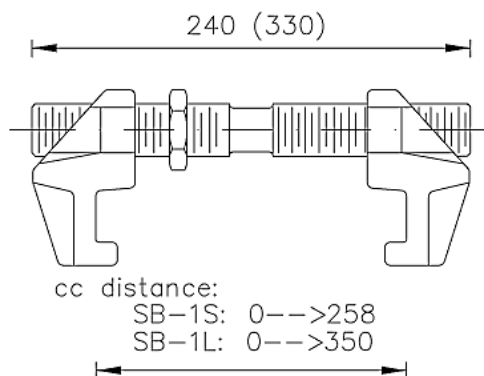
SB-1
