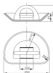
FLUSH
