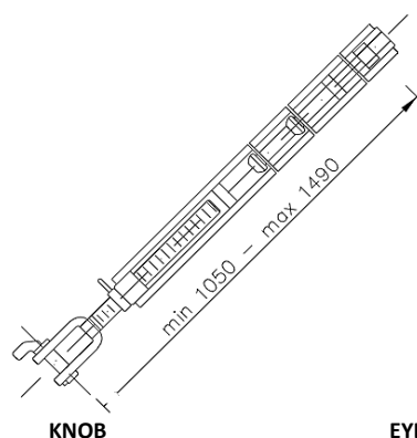
KNOB
