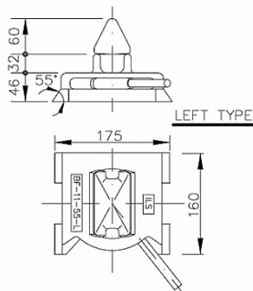
LONGITUDINAL 55°
