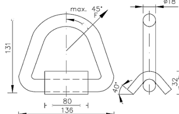
20 TON
