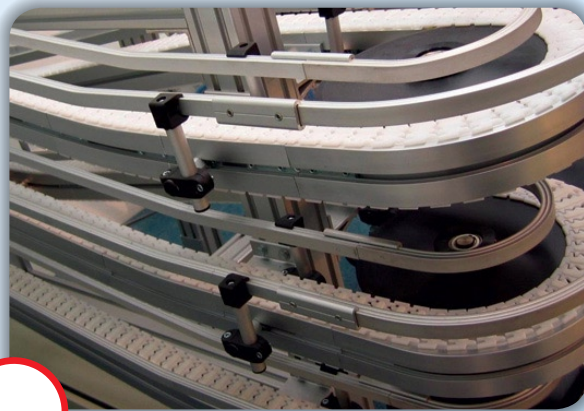
Alpinbuffer til niveauændring eller blot som buffer.
