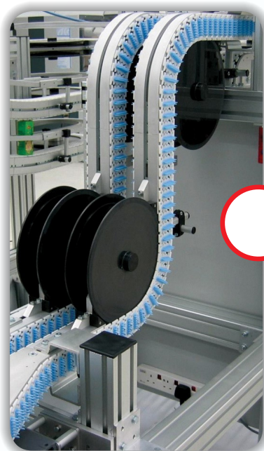
Klemelevator til lodret løft i ét kontinuerligt flow.
