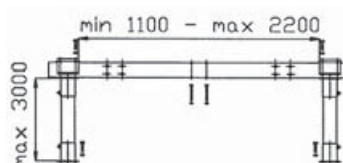
Art.nr. 7195. Bredt gulvstativ til bigbag/ container.
