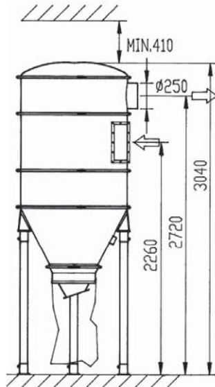
F30000 med ekstra modulring
