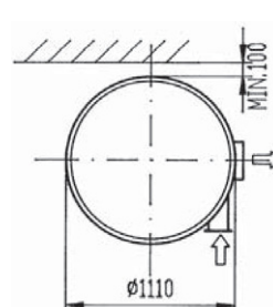
F30000 set fra oven
