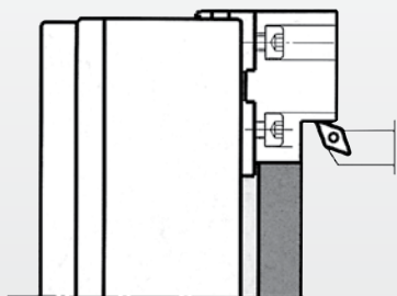
Utvändig uppspänning
