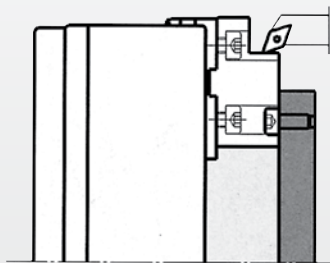
Invändig uppspänning
