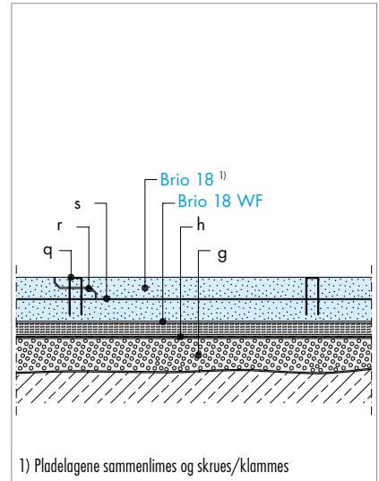
GB 6 Flerlagskonstruktion
