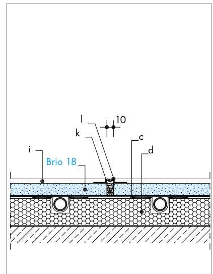
GB 3 Bevægelsesfuge
