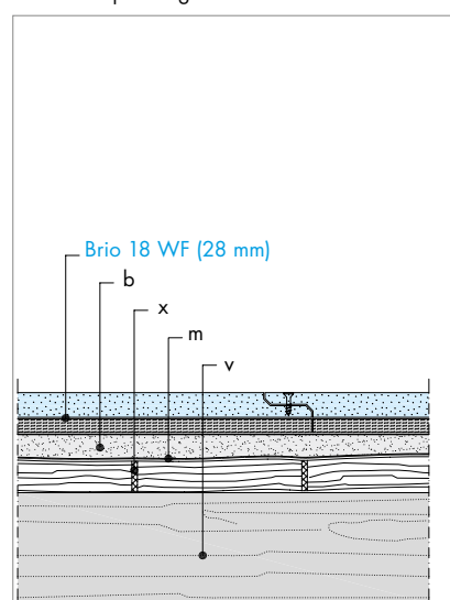
GB 9 Træbjælkelag
