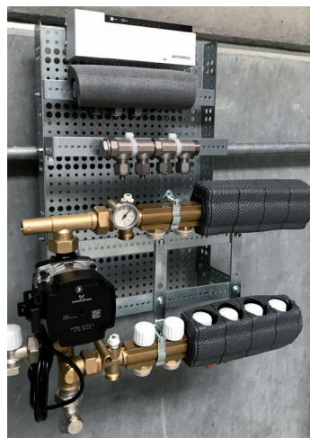
BUNDMODUL med 6 kredse gulvvarme. 3 varme og 4 kolde kredse brugsvand + styring og isolering.
