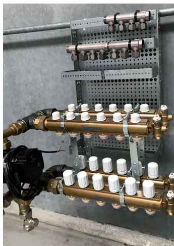
BUNDMODUL med 2x6 kredse gulvvarme. 4 varme og 7 kolde kredse brugsvand. Vinklet shunt.
