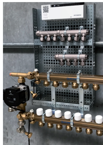
BUNDMODUL med 7 kredse gulvvarme. 7 kolde og 4 varme kredse brugsvand + gulvvarmestyring.
