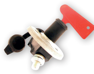
Batteribrytare 100 A, 12/24 V, 500 A - 10 sek. Med plastnyckel och dammskydd. Monteras med 2 skruv/bult, hål. Artikelnr: 16-328625
