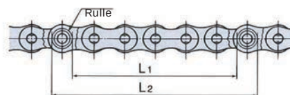
Måling af afstand mellem rullerne
