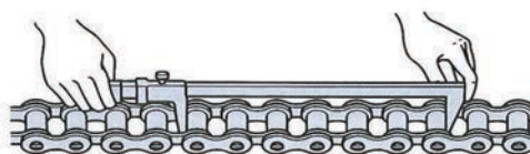
Placering af skydelære ved måling over 6 led
