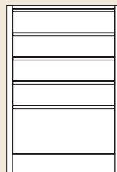
BE-600-4/S-1/M Sektion med 5 lådor. Lådstorlek x 4 B 495 x H 100 x D 600mm. Lådstorlek x 1 B 495 x H 220 x D 600mm. Modulstorlek B 600 x H 880 x D 660mm.
