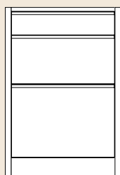
BE-600-1/S-1/M-1/L Sektion med 3 lådor Lådstorlek x 1 B 495 x H 100 x D 600mm. Lådstorlek x 1 B 495 x H 220 x D 600mm. Lådstorlek x 1 B 495 x H 360 x D 600mm. Modulstorlek B 600 x H 880 x D 660mm.
