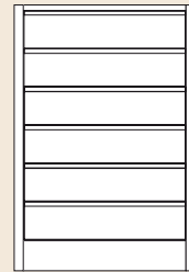
BE-600-6/S Sektion med 6 lådor. Lådstorlek x 6 B 495 x H 100 x D 600mm. Modulstorlek B 600 x H 880 x D 660mm.
