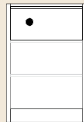
BE-600-Paper Sektion med 3 lådor. Låda för centrummatad pappersrulle. B 495 x H 220 x D 600mm. Passar i modulstorlek B 600 x H 880 x D 660mm.
