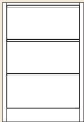
BE-600-3/M Sektion med 3 lådor. Lådstorlek x 3 B 495 x H 220 x D 600mm. Modulstorlek B 600 x H 880 x D 660mm.
