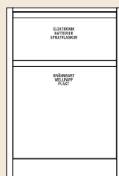
BE-600-2x/Miljö Sektion med 2 lådor. Lådstorlek x 1 B 495 x H 220 x D 600mm. Lådstorlek x 1 B 495 x H 490x D 600mm. Modulstorlek B 600 x H 880 x D 660mm.
