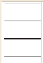
BE-600-2/S-2/M Sektion med 4 lådor Lådstorlek x 2 B 495 x H 100 x D 600mm. Lådstorlek x 2 B 495 x H 220 x D 600mm. Modulstorlek B 600 x H 880 x D 660mm.
