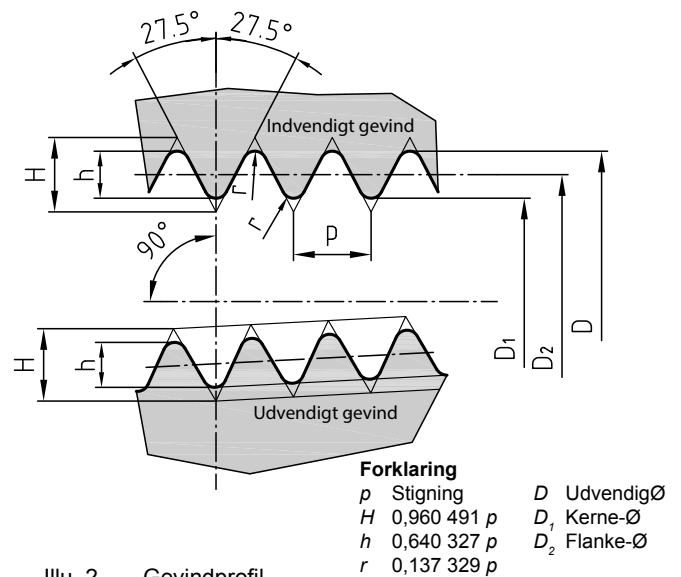
Illu. 2 Gevindprofil
