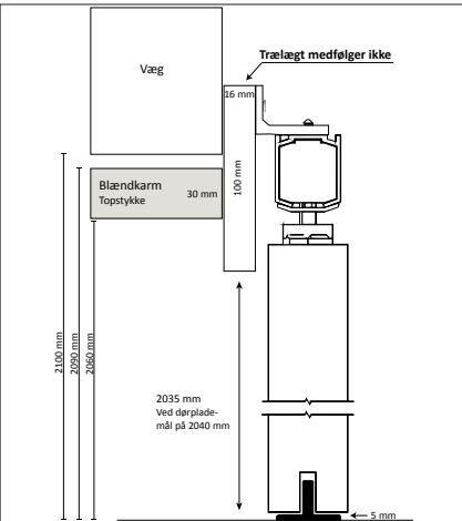
Opsætning af skydedør uden kappe
