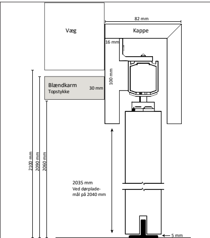
Opsætning af skydedør med kappe
