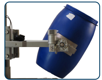
Drivet klämverktyg för tilt av fat/rollar
