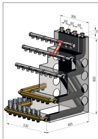
Max. bestykning af et BUNDMODUL for at det kan være i et 60 cm skab. 12 gulvvarme-, 16 koldtvars- og 9 varmtvandskredse.
