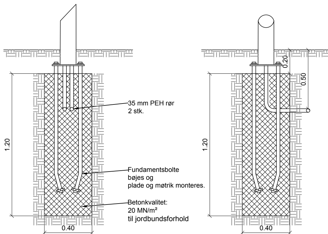
Detailplan fundament for 7 og 8 meter Rundkonisk master
