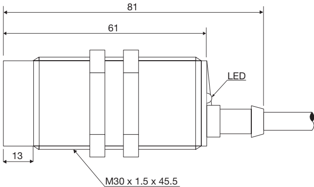
Fig. 7 Kabel CA30CAN...A2IO
