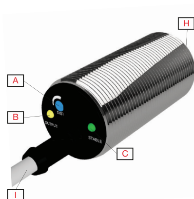
Fig. 1 CA30 Kabel
