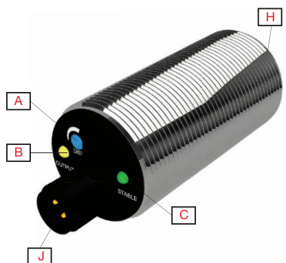
Fig. 2 CA30 Stik
