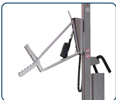
Rullexpander för att lyfta och rotera rollen 90°
