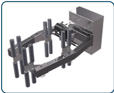
Drivet klämverktyg för vridning av fat/rullar
