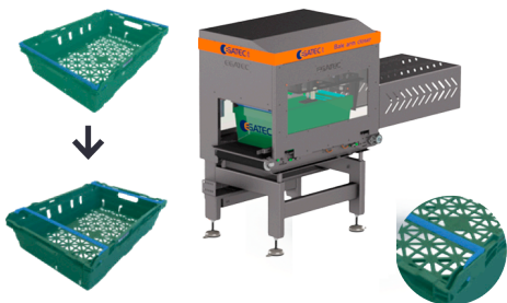
EGAbale Arm Closer
