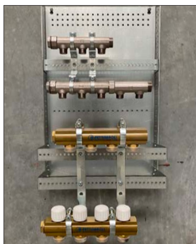
Skaktløsning med 4 gulvvarme-, 5 koldtvands- og 3 varmtvandskredse.
