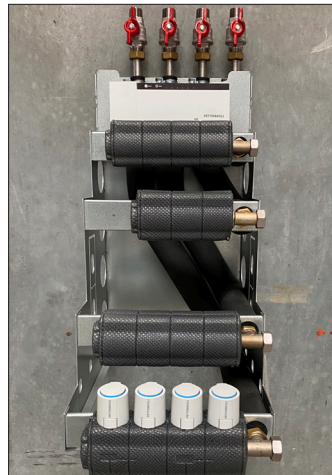
Eksempler på BUNDMODULER Model TM og S. Specialkonstruktion mht. antal kredse samt tilbehør såsom ventiler, gulvvarmestyring og telestater.
