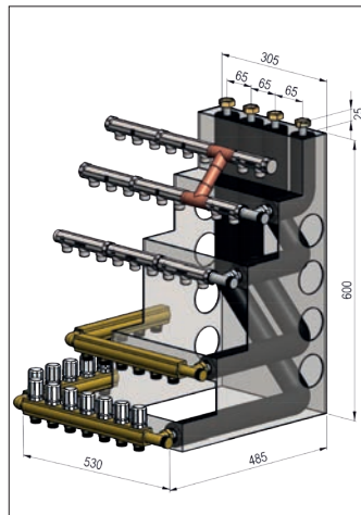
Max. bestykning af et BUNDMODUL for at det kan være i et 60 cm skab. 12 gulvvarme-, 16 koldtvands- og 9 varmtvandskredse.
