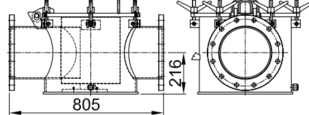
DN 250
