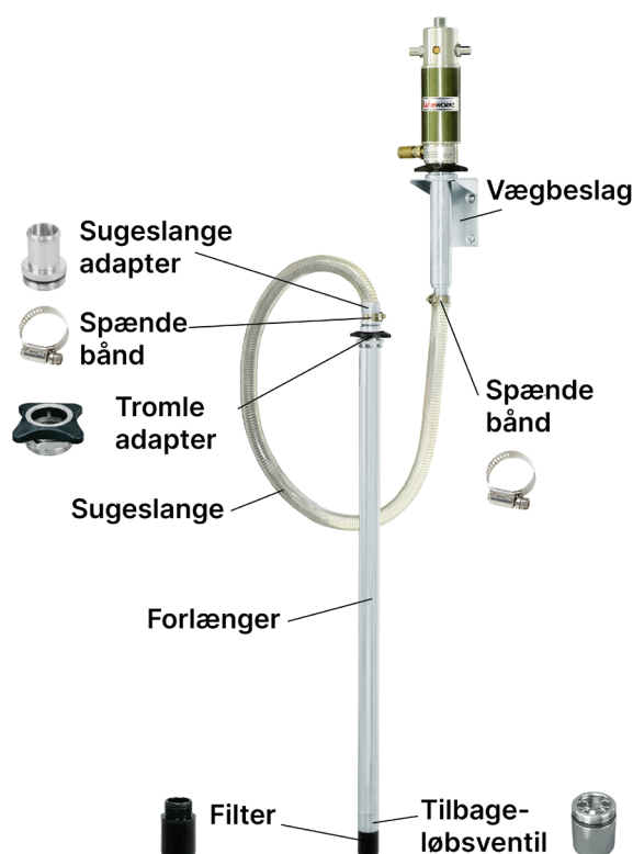
7200-WB10000 Vægadapter til pumpe. Passer til 60 - 208 ltr. tromle.
