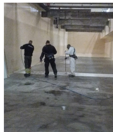
Påføring av glassfiberbelegg, Ladehammeren renseanlegg
