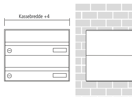
Montering med skyggefuge
