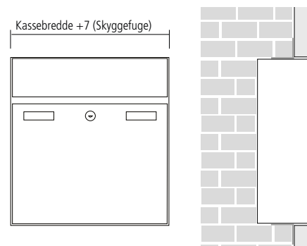
Montering med skyggefuge (ideel til facader med udhæng)
