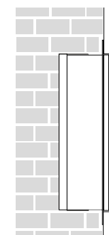
Montering med skyggefuge (ideel til facader med udhæng)
