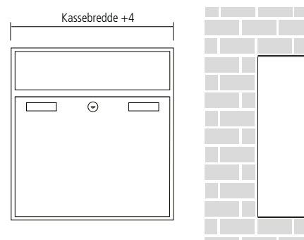
Montering med skyggefuge (ideel til facader med udhæng)
