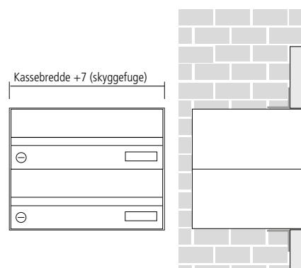
Montering med skyggefuge
