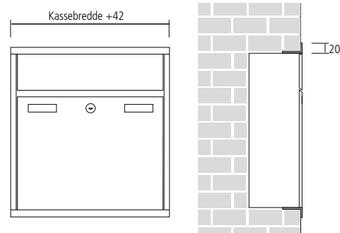
Planforsænket indbygning med tætsiddende beklædning
