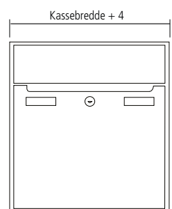
Planforsænket indbygning med tætsiddende beklædning
