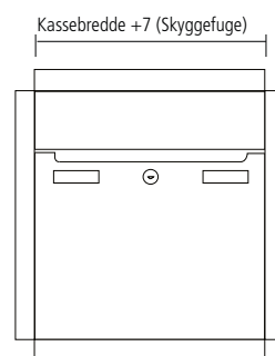
Montering med skyggefuge (ideel til facader med udhæng)
