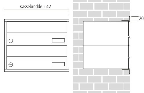
Planforsænket indbygning med tætsiddende beklædning
