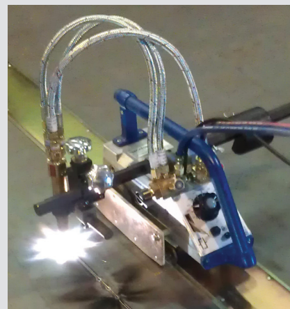
Gasskärning används för delning av plåten.
