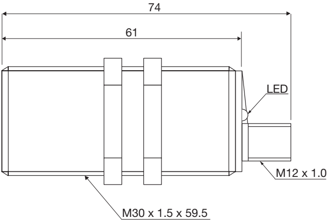
Fig. 8 Stik CA30CAF...M1IO
