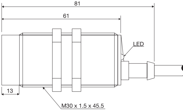
Fig. 7 Kabel CA30CAN...A2IO
