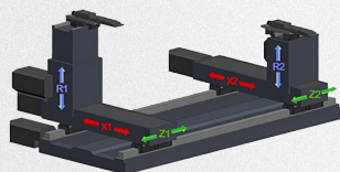
Pladeanslag system op til 6-akset
