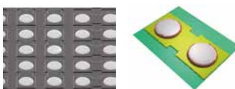
Halvledartestmönster (TEG)
